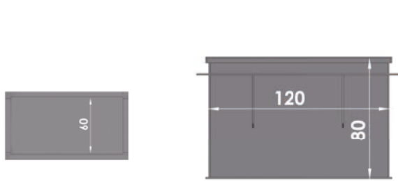
Technikschacht für Gegenstromanlage
