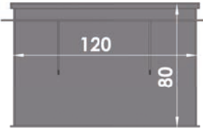
Pozo tecnológico para el chorro contracorriente
